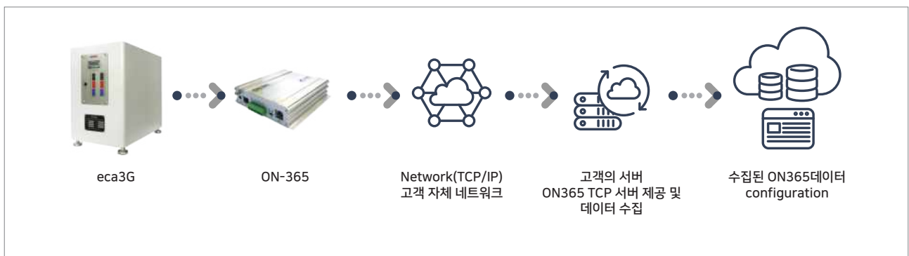
[그림-2] 독립망 사용고객용 실시간 낙뢰방호 모니터링 서비스 구성도
