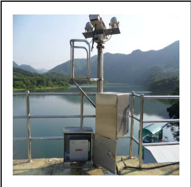
공사설명 4. 댐저수위 감시카메라 장비설치
