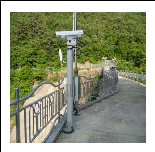
공사설명 5. 괴산댐 하류영상 카메라
