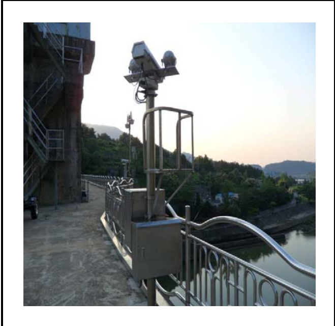
공사설명 6. 공도교 끝 발전방류 감시카메라 합체설치
