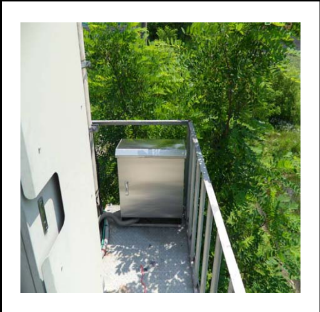
공사설명 10. 방류예경보 제3국 함체설치
