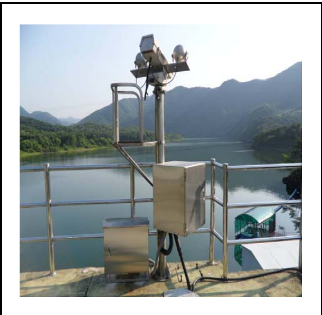
공사설명 4. 댐저수위 감시카메라 합체설치
