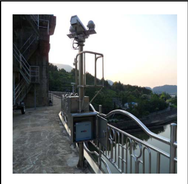
공사설명 6. 공도교 끝 발전방류 감시카메라 장비설치
